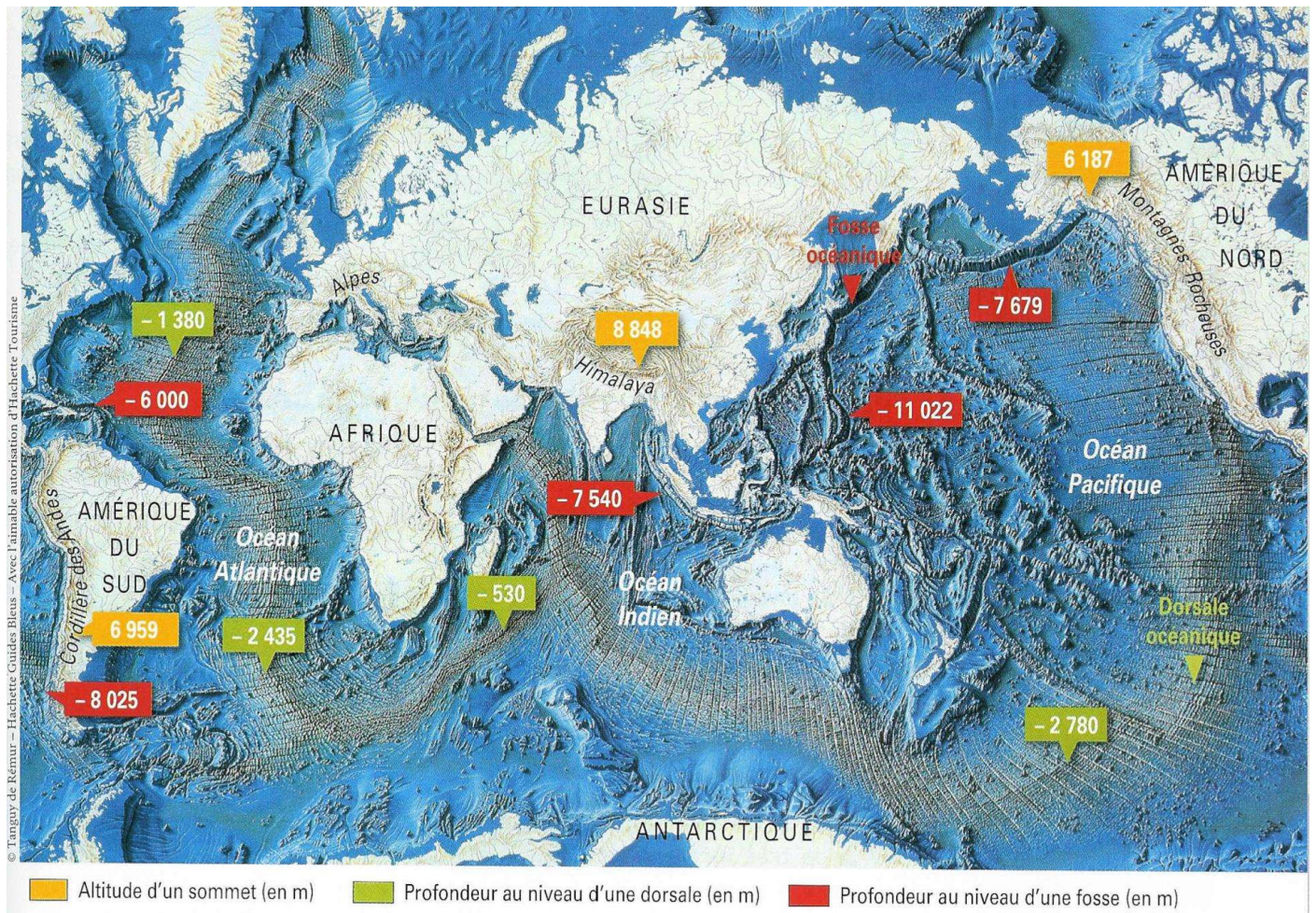
Carte des reliefs terrestres
