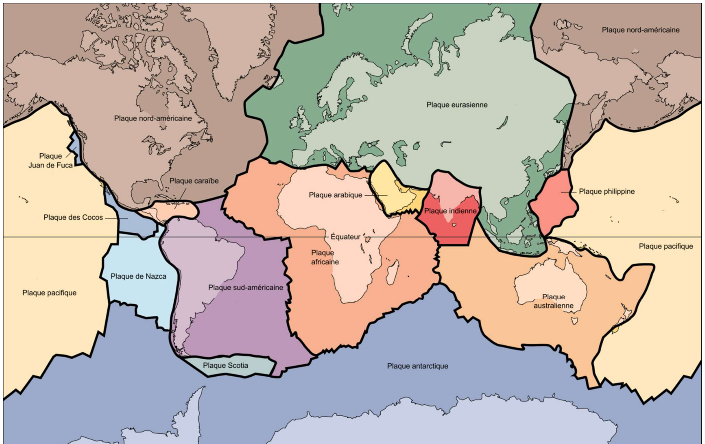
Carte des plaques tectoniques
